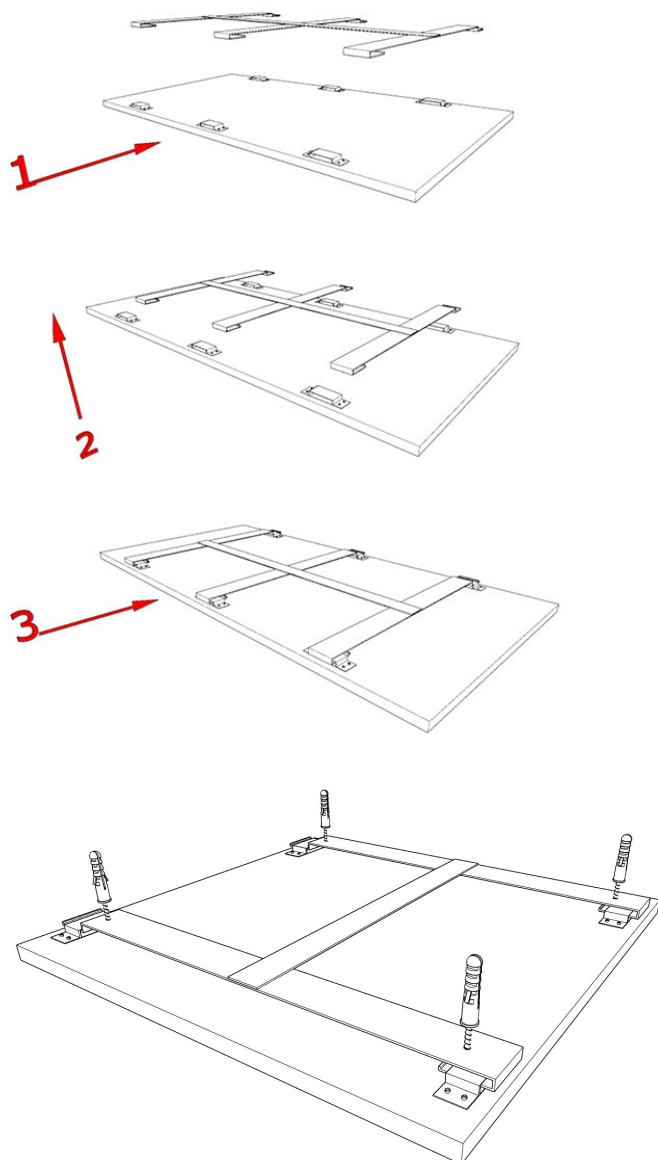
Montaż na ramce Rys.1
